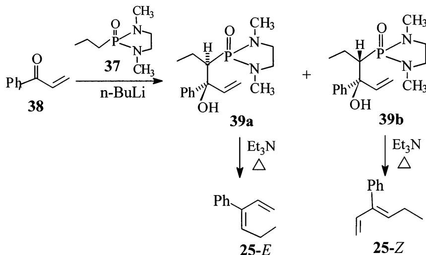
Scheme 18.
