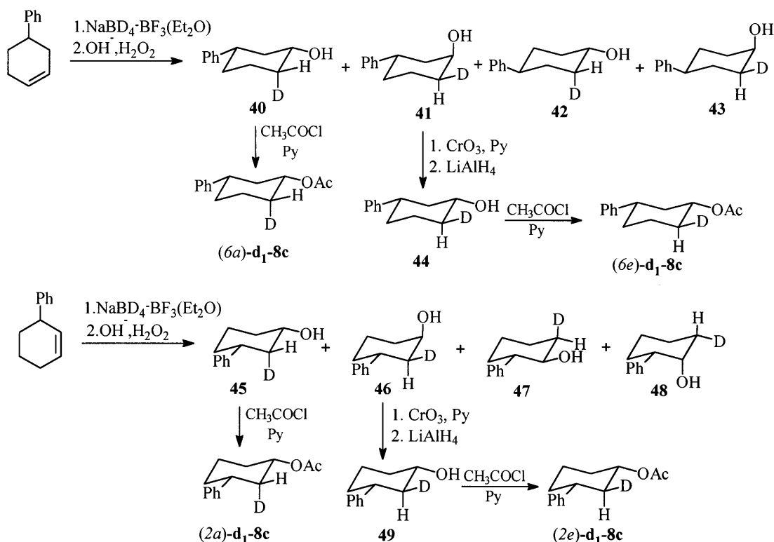
Scheme 20.
