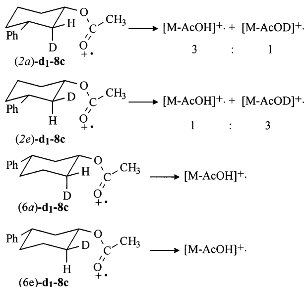
Scheme 14.
