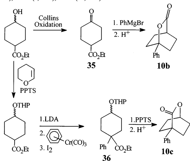
Scheme 17.
