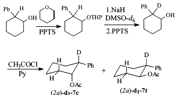
Scheme 19.
